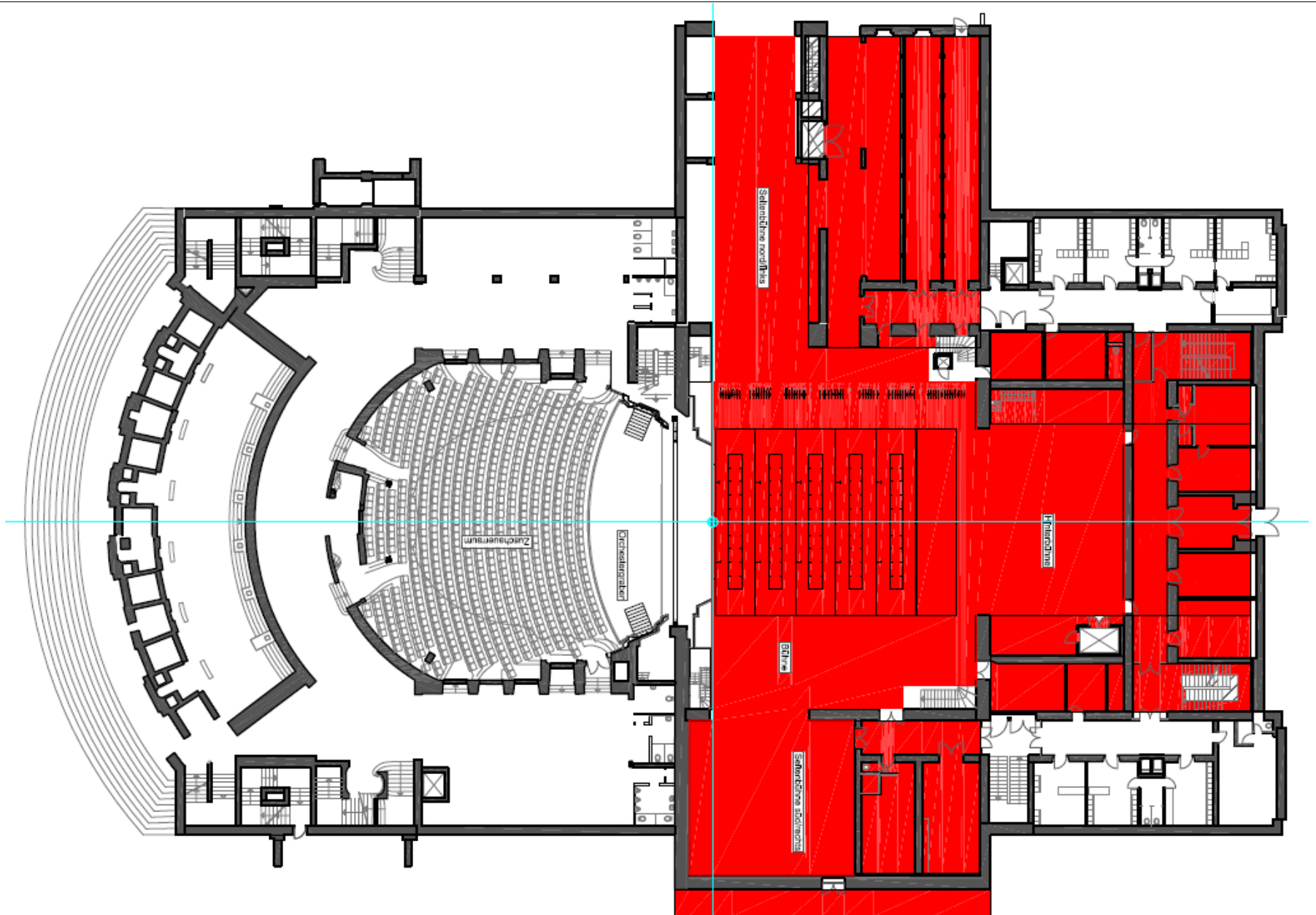
Grundriss Opernhaus Stuttgart (NEU)
